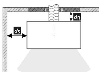
Hátsó kéménycsatlakozás
